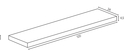
GRADINO PLUS ANGOLARE SX** 34x120x4,5 cm Rect - 13 3/8 "x48"x1 3/4 " NATURALE ± 9,5 mm
